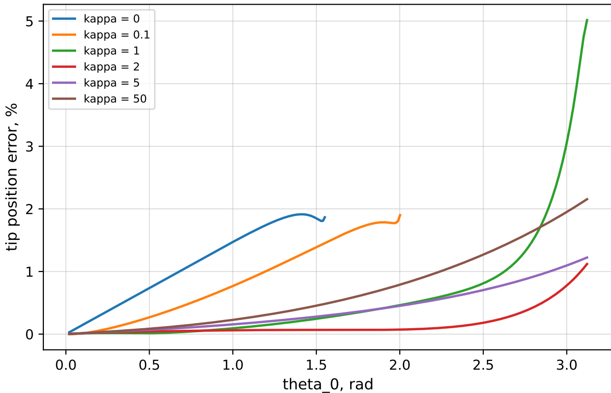
PRB 3R Tip Position Error
